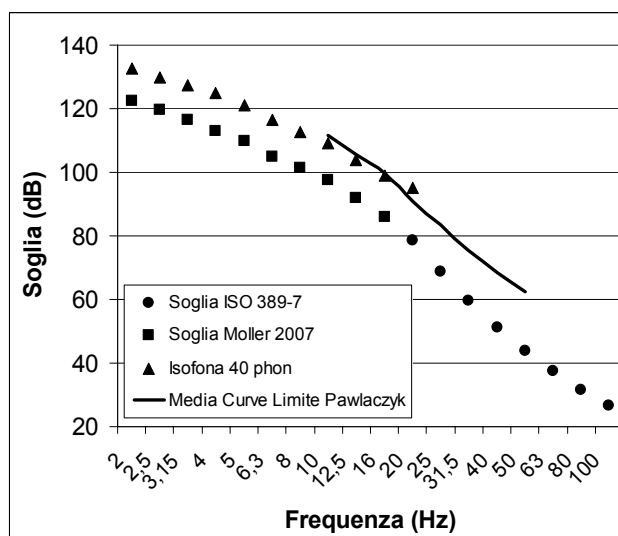
Figura 7 – Alcune curve rilevanti per la valutazione dell'esposizione ad infrasuoni
