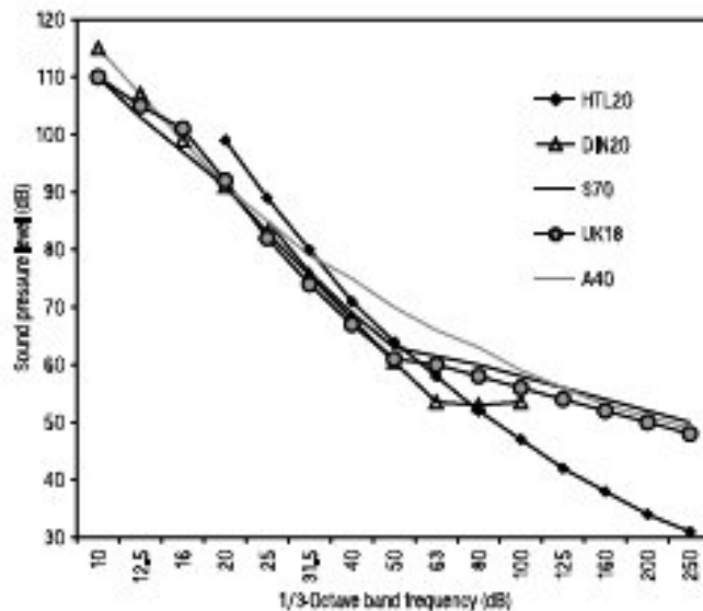
Figura 6 – Determinazioni della soglia di tollerabilità per onde sonore di bassa frequenza a partire da curve limite nazionali
