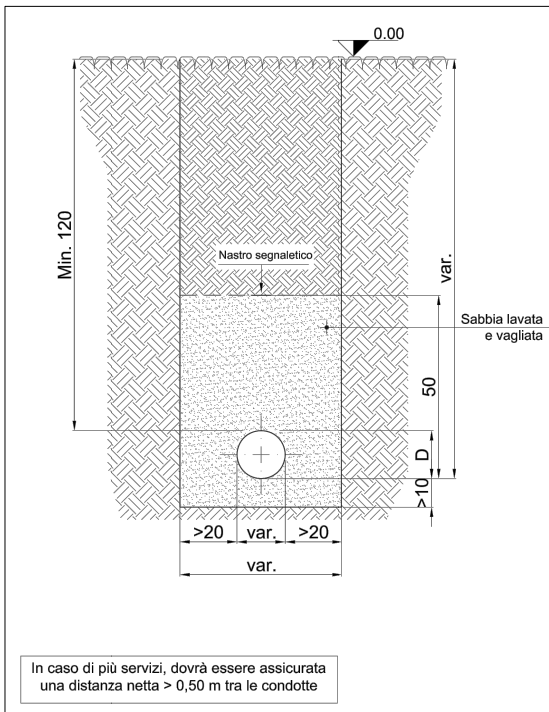
SCHEMA TIPO DI ESECUZIONE SCAVO IN TERRENO NATURALE PER POSA ACQUEDOTTO
