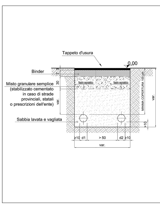
SCHEMA TIPO DI ESECUZIONE SCAVO SU SEDE STRADALE ASFALTATA PER POSA DI DUE CONDOTTE (ACQUEDOTTO E ALTRO SERVIZIO)
