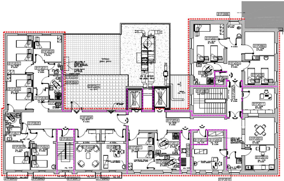
Figura 2. Planimetria OSCO
